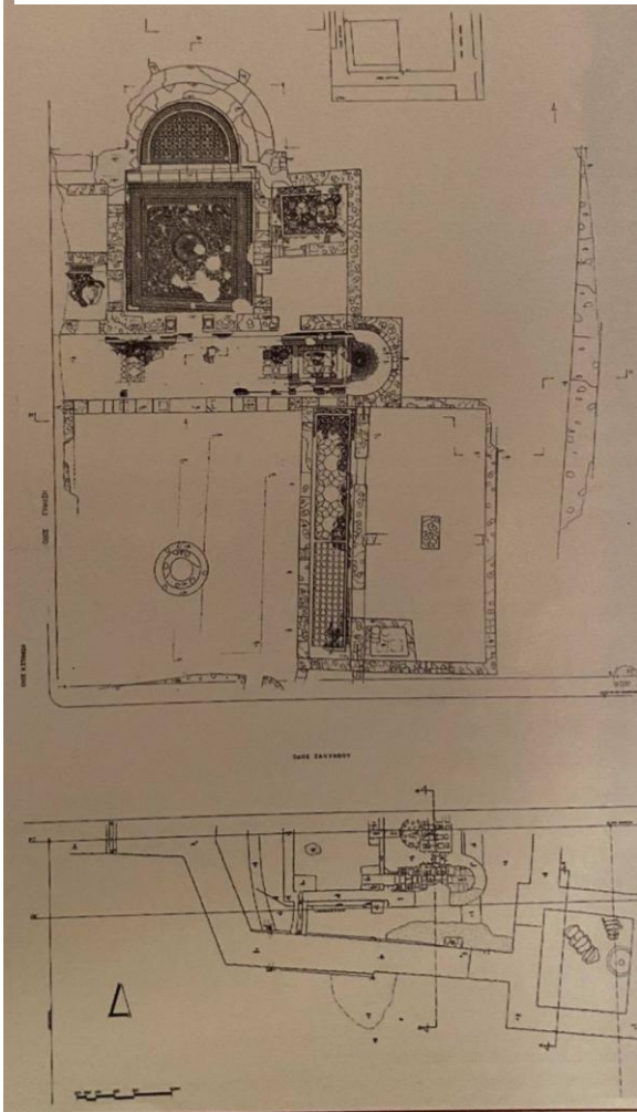
Εικόνα 7: Η κατοψη της έπαυλης
