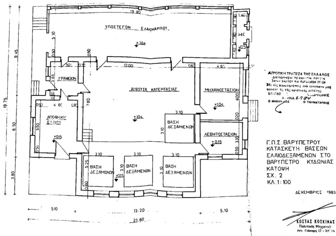
Εικόνα 3: Σχέδιο κατασκευής βάσεων ελαιοδεξαμενών | Φ217
