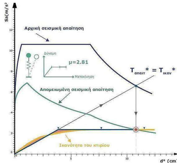
Σχήμα 5.9 «Διάγραμμα προσδιορισμού της στοχευόμενης μετακίνησης EC8-3»
