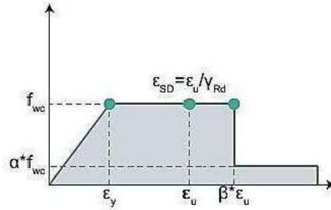
Σχήμα 5.13 «Σκελετικό διάγραμμα τάσεων – ανηγμένων παραμορφώσεων»
