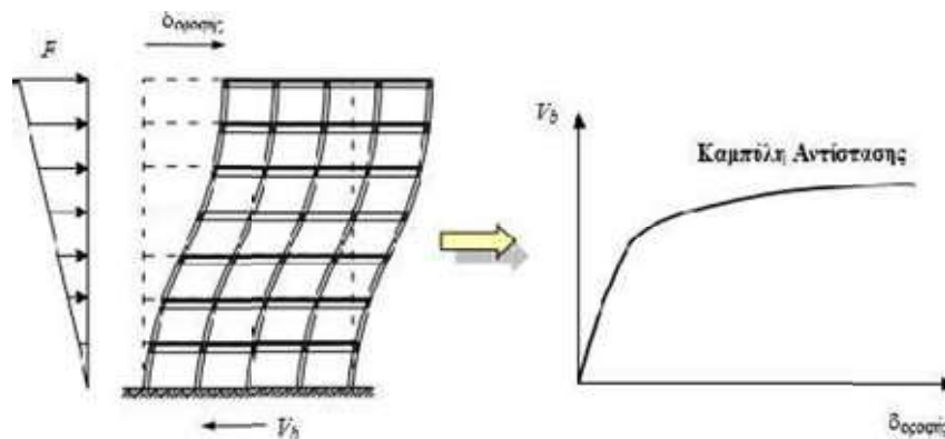
Σχήμα 4.3 «Καμπύλη τέμνουσας βάσεως – μετακίνησης (V-δ) για μη γραμμική στατική ανάλυση υπό σταδιακώς αυξανόμενη ένταση. (Ρεπαπής, 2007)»
