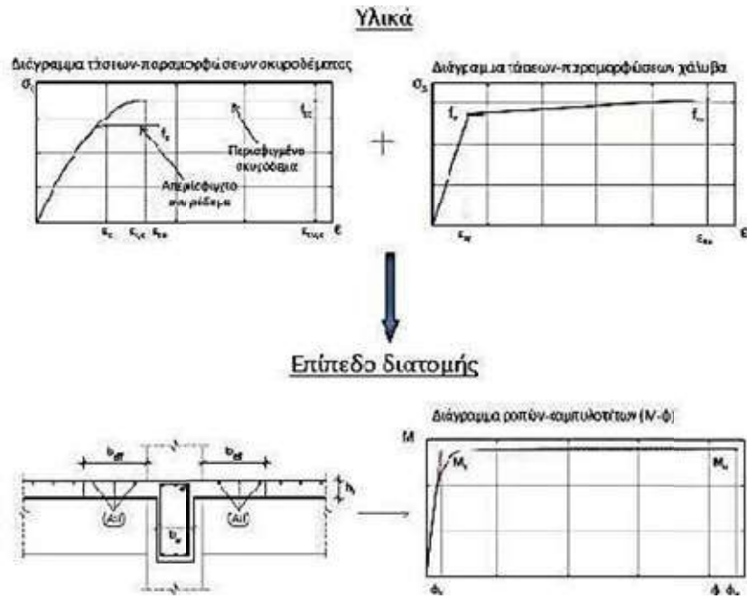
Σχήμα 5.2 «Διαγραμματική ροή ανάλυσης Pushover σε επίπεδο διατομής κατά HoloBim»
