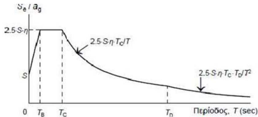
Σχήμα 3.1 «Γενική μορφή ελαστικού φάσματος απόκρισης ψευδοεπιταχύνσεων»
