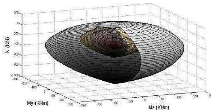
Σχήμα 5.6 «Τρισδιάστατη απεικόνιση διαγραμμάτων αλληλεπίδρασης διαξονικής κάμψης- αξονικής δύναμης»
