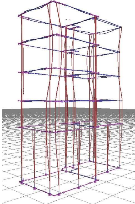
Σχήμα 7.0 «Ιδιόμορφη ταλάντωση του φορέα»
