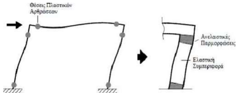
Σχήμα 4.4 «Θέσεις πιθανών πλαστικών αρθρώσεων σε μέλη απλής κατασκευής υπό σεισμική ένταση»
