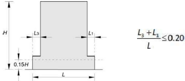
Σχήμα 3.3 «Μεμονωμένη εσοχή σε υψος μεγαλύτερο του 15% του συνολικού»
