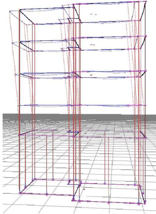
Σχήμα 7.3 «2 η ιδιομορφή ταλάντωσης φορέα κατά την διεύθυνση ζ-ζ'»
