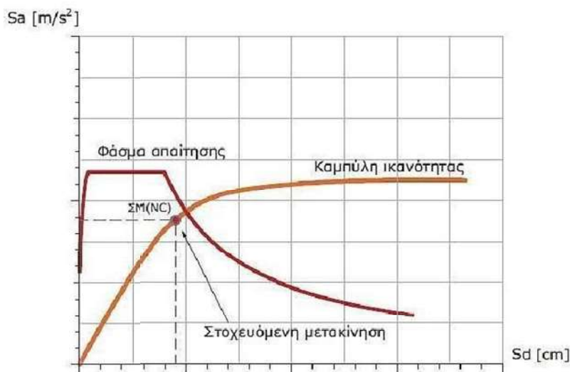
Σχήμα 5.8 «Διάγραμμα απαίτησης ικανότητας»
