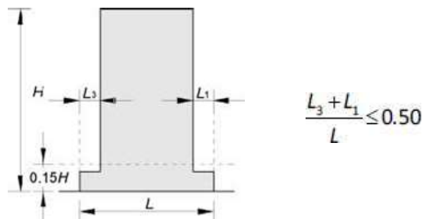
Σχήμα 3.4 «Μεμονωμένη εσοχή σε ύψος μικρότερο του 15% του συνολικού»
