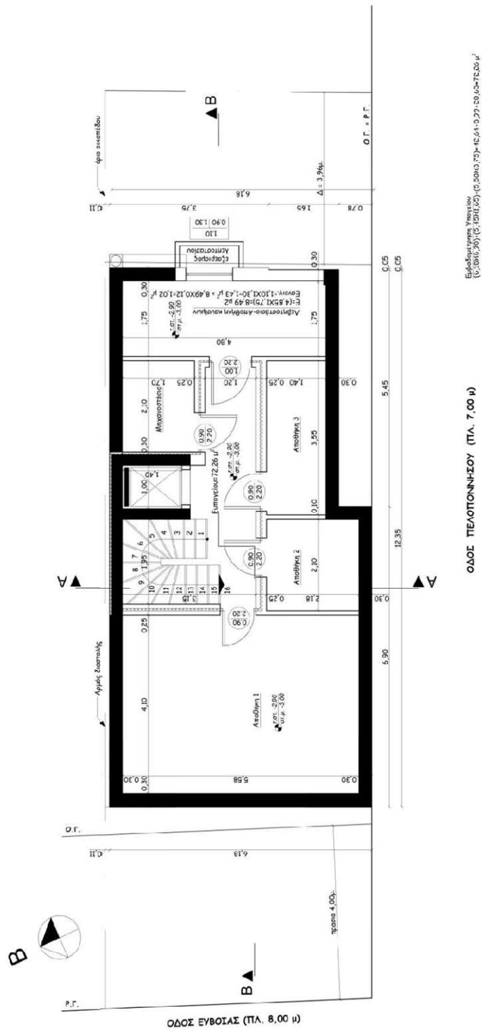
Σχήμα 1.1: «Κάτοψη Υπογείου»
