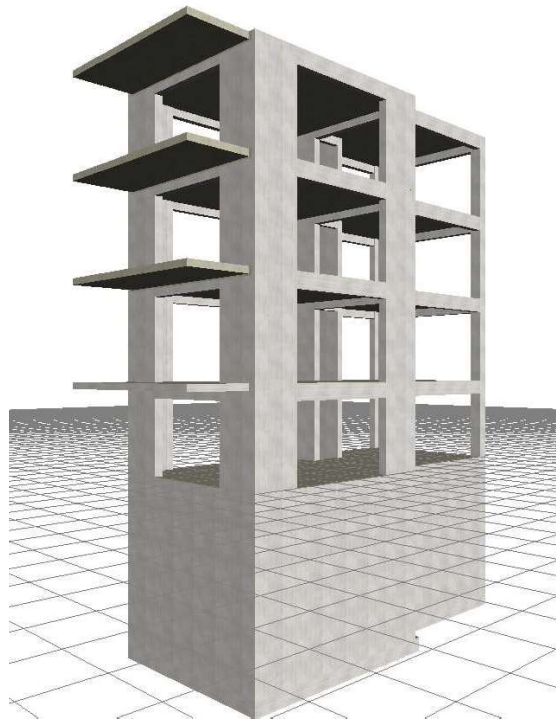
Σχήμα 6.1 «Τρισδιάστατη απεικόνιση φέροντα οργανισμού κτιρίου»
