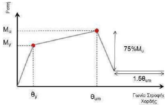
Σχήμα 5.4 «Γενική μορφή διαγράμματος M-\theta »
