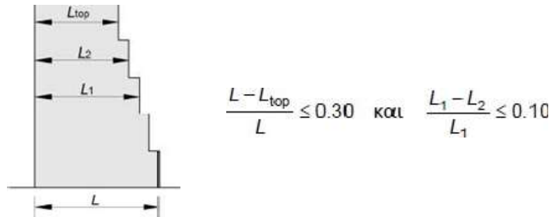
Σχήμα 3.5 «Εσοχές που παραβιάζουν την κατακόρυφη συμμετρία»
