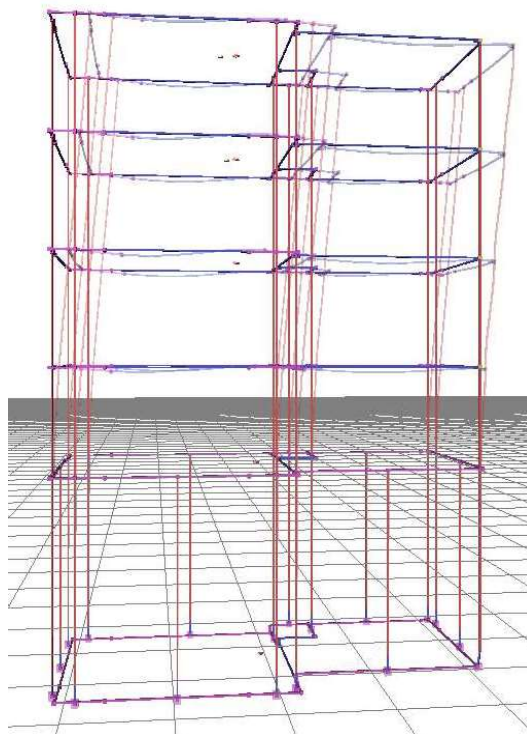
Σχήμα 6.8 «1 η ιδιομορφή ταλάντωσης φορέα κατά την διεύθυνση χ-χ»
