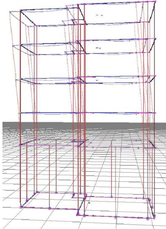
Σχήμα 6.9 «2 η ιδιομορφή ταλάντωσης φορέα κατά την διεύθυνση ζ-ζ»
