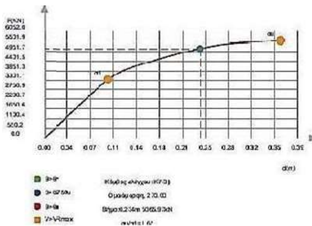
Σχήμα 5.1 «Διάγραμμα καμπύλης αντίστασης Δύναμης –Μετακίνησης»
