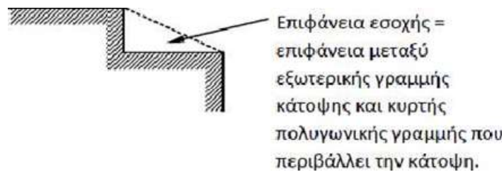
Σχήμα 3.1 «Καθορισμός επιφάνειας εσοχής ορόφου»
