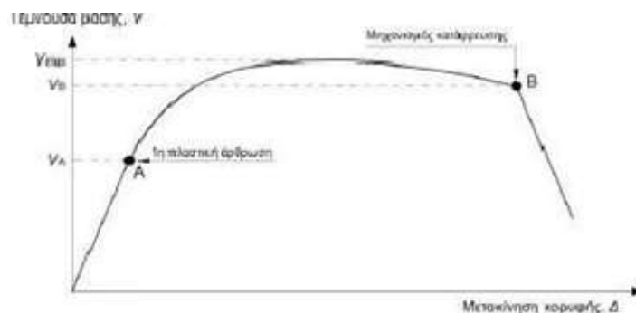
Σχήμα 3.2 «Υπολογισμός λόγου au/a1 εάν είναι διαθέσιμη η καμπύλη ικανότητας»
