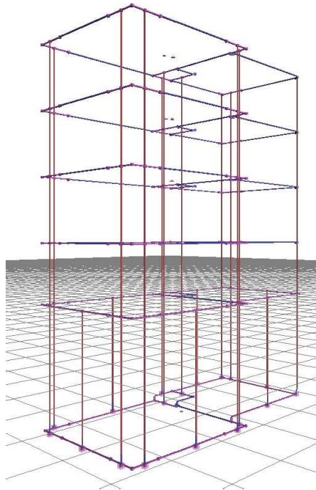
Σχήμα 6.7 «Μαθηματικό προσομοίωμα με πρόβλεψη»
