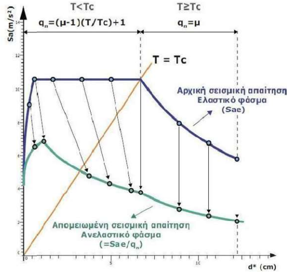
Σχήμα 5.11 «Διάγραμμα απομείωσης της σεισμικής απαίτησης q_n ( S_a = S_{ae}/q_n )»
