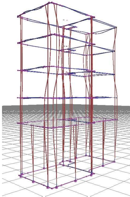
Σχήμα 7.4 «Ιδιόμορφη ταλάντωση του φορέα»
