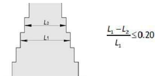
Σχήμα 3.2 «Βαθμιδωτές εσοχές που δεν παραβιάζουν την αξονική συμμετρία»
