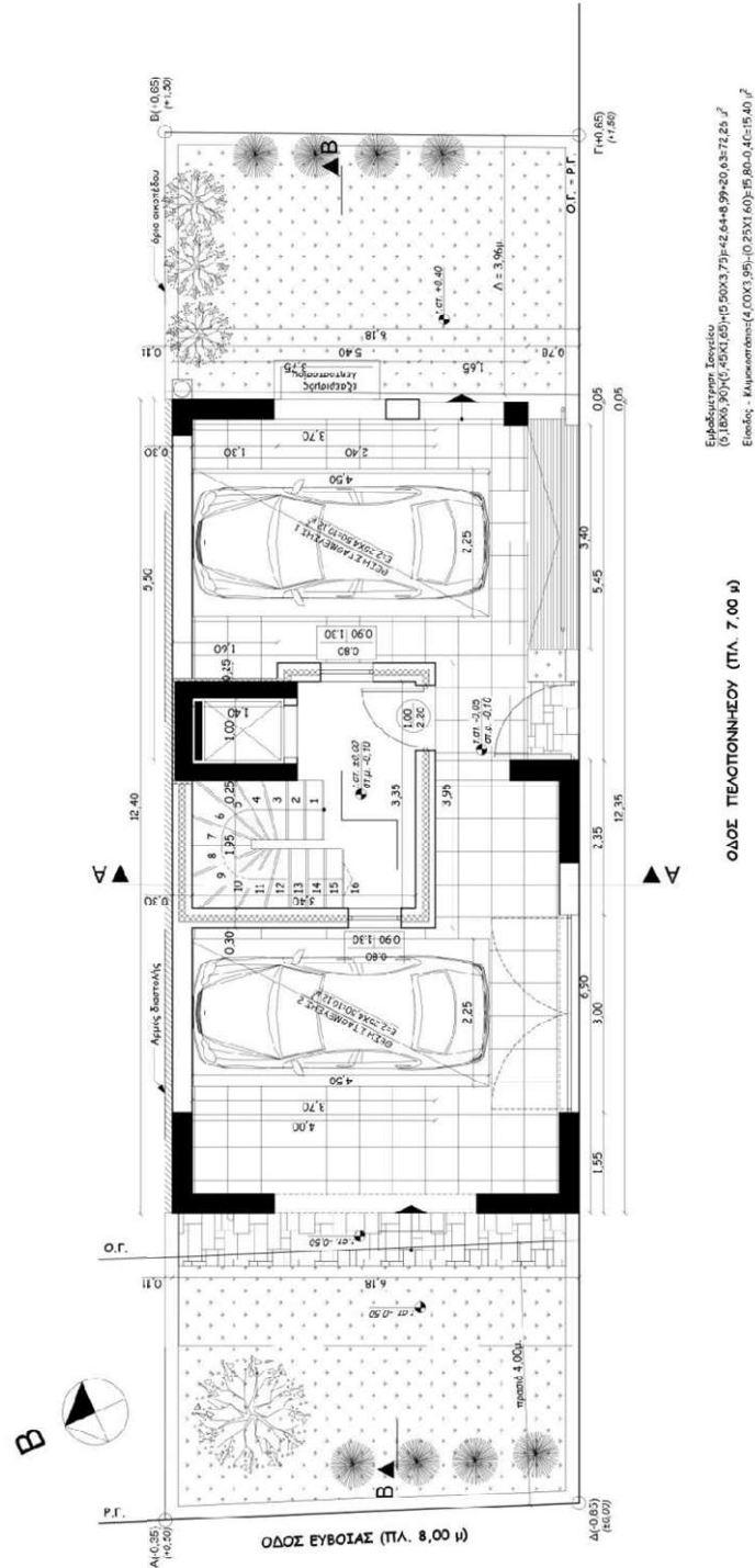
Σχήμα 1.2: «Κάτοψη Ισογείου»
