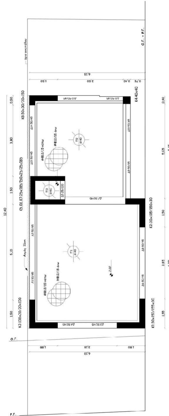
Σχήμα 6.1 «Ξυλότυπος Θεμελίωσης»
