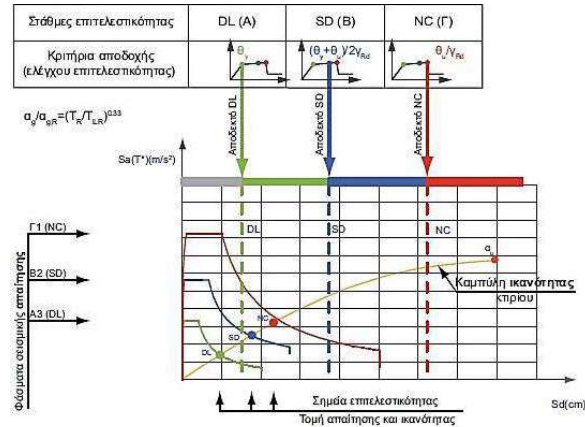
Σχήμα 5.10 «Κριτήρια αποδοχής – ελέγχου επιτελεστικότητας»
