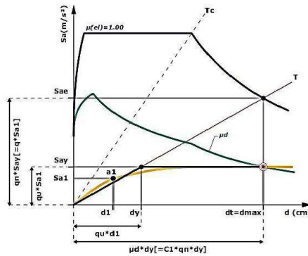
Σχήμα 5.12 «Διάγραμμα ADRS ( S_a-d ). Τεκμηρίωση των q , q_n , q_u »
