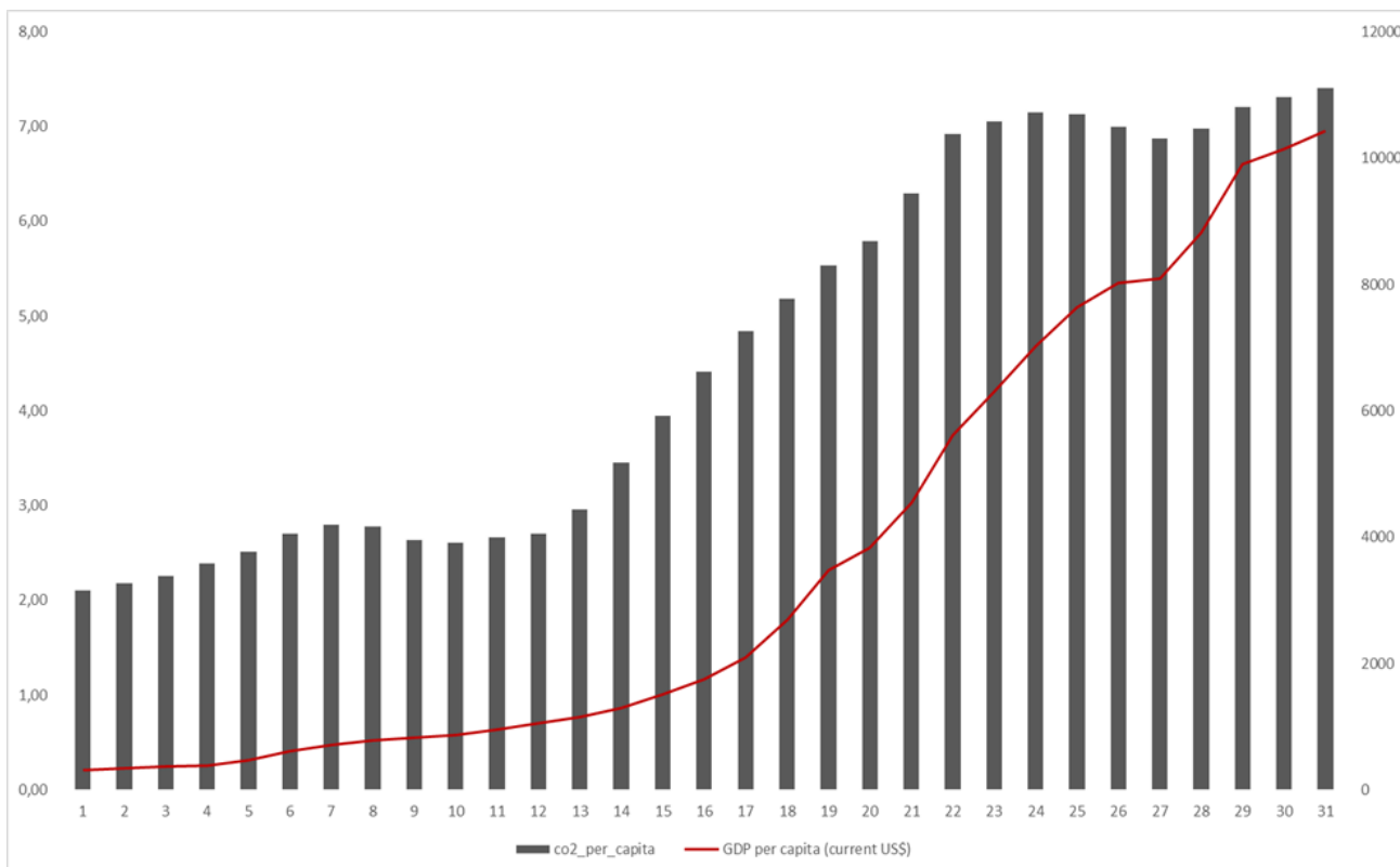
Γράφημα 2: 3.2: Εκπομπές CO2 και Α.Ε.Π. κατά κεφαλήν ( https://www.worldbank.org )
