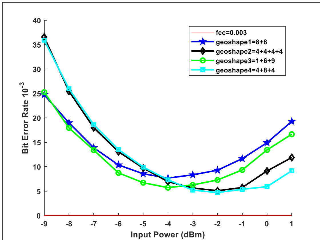
Εικόνα 54: Γραφική παράσταση BER συνάρτηση της ισχύος εισόδου για απόσταση 20 spans στα 75 GHz για τους 4 διαφορετικούς αστερισμούς με RRC.
