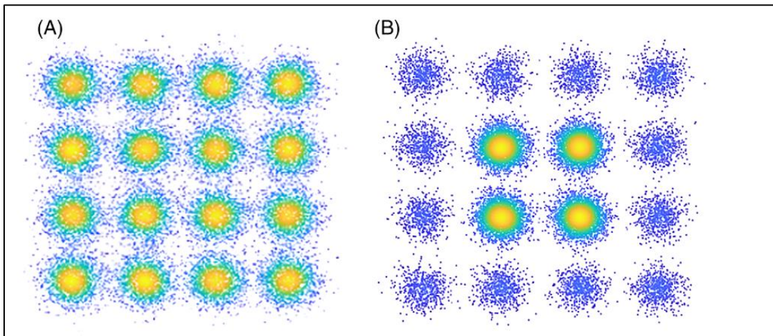
Εικόνα 37: (A)Τυπική 16-QAM διαμόρφωση (B)16QAM πιθανοκρατική διαμορφωση. [13]
