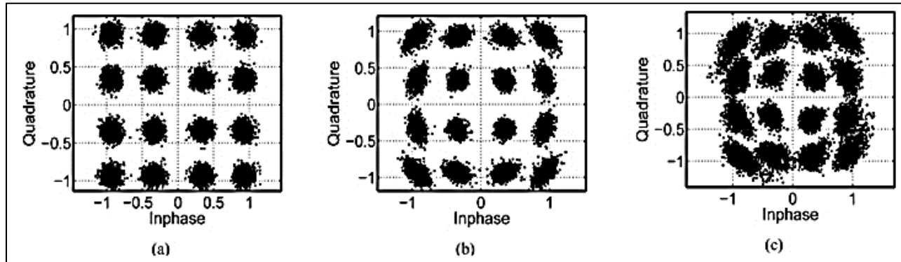
Εικόνα 34: (α)16QAM αστερισμός χωρίς την παρουσία μη γραμμικών φαινομένων.(β) Εμφανή επίδραση μη γραμμικών φαινομένων στα ακριανά σύμβολα λόγω της μεγαλύτερης ισχύος που υφίστανται με αποτέλεσμα το ωειδές σχήμα που απεικονίζεται (που σημαίνει αλλαγή στην φάση) .(c) Περεταίρω αύξηση των μη γραμμικών φαινομένων με αποτέλεσμα την καταστροφή του σήματος.
