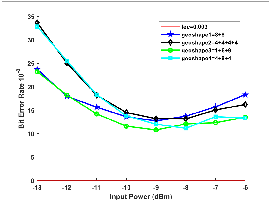
Εικόνα 50: Γραφική παράσταση BER συνάρτησης της ισχύος εισόδου για απόσταση 20 spans στα 50 GHz για τους 4 διαφορετικούς αστερισμούς.
