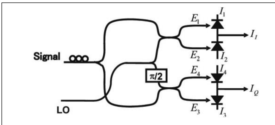
Εικόνα 22: Διαμόρφωση του ομόδунου δέκτης ποικίλων φάσεων με χρήση ενός οπτικού υβρίδιου 90^\circ . Η συνιστώσα I (in-phase) και η συνιστώσα Q (quadrature) του σήματος μιγαδικού πλάτους λαμβάνονται ταυτόχρονα. [2]
