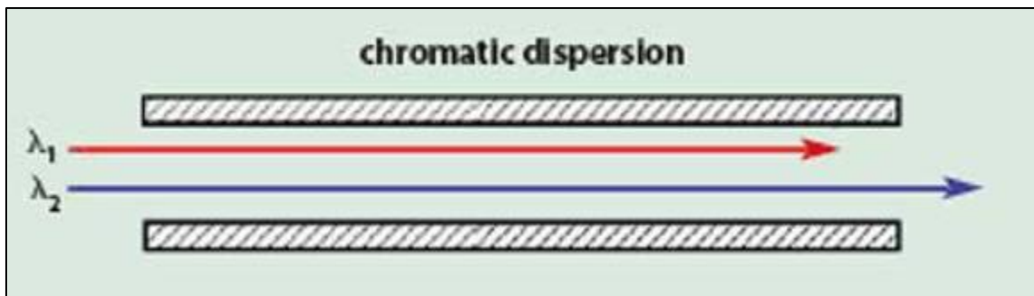
Εικόνα 5: Χρωματική διασπορά. [18]
