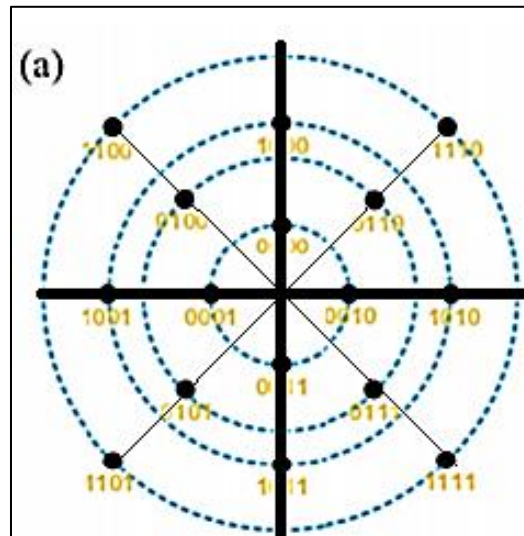
Εικόνα 43: Αναπαράσταση του αστερισμού 16=4+4+4+4 . Με έντονο χρώμα γίνεται η τομή των κύκλων ανά γωνίες \theta_1=90^\circ ενώ με το πιο μικρές μαύρες ευθείες γίνεται η τομή των κύκλων ανά γωνίες \pi/4=45^\circ . Έτσι έχοντας τις γωνίες καθώς και τις ακτίνες προσδιορίζουμε ακριβώς το σημείο που θα βάλουμε τα σύμβολα μέσω του MATLAB για να έχουμε τον παραπάνω αστερισμό.
