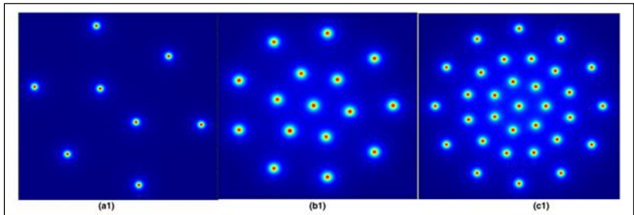
Εικόνα 36: Παραπάνω βλέπουμε κάποιους αστερισμούς δακτυλίου για GS-8-QAM,GS-16-QAM,GS-32-QAM αντίστοιχα. Κάθε σύμβολο έχει ίδια πιθανότητα εμφάνισης και για κάθε QAM αντίστοιχα βλέπουμε πως τοποθετούνται για να επιτευχθεί ένα καλύτερο αποτέλεσμα και να περιοριστούν όσο γίνεται τα μη γραμμικά φαινόμενα. [1]
