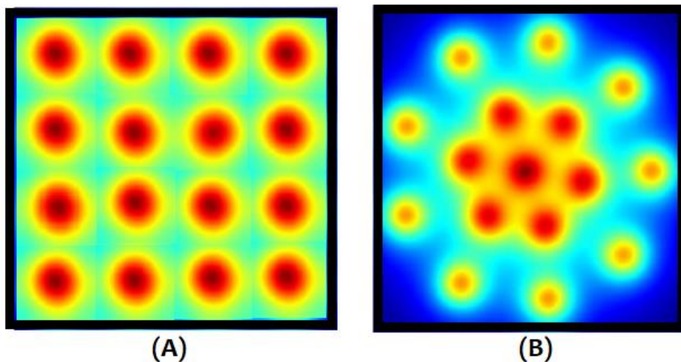
Εικόνα 38: (A) Τυπική 16-QAM διαμόρφωση (B) Συνδυασμός πιθανοκρατικής και γεωμετρικής διαμόρφωσης για 16-QAM. [1]
