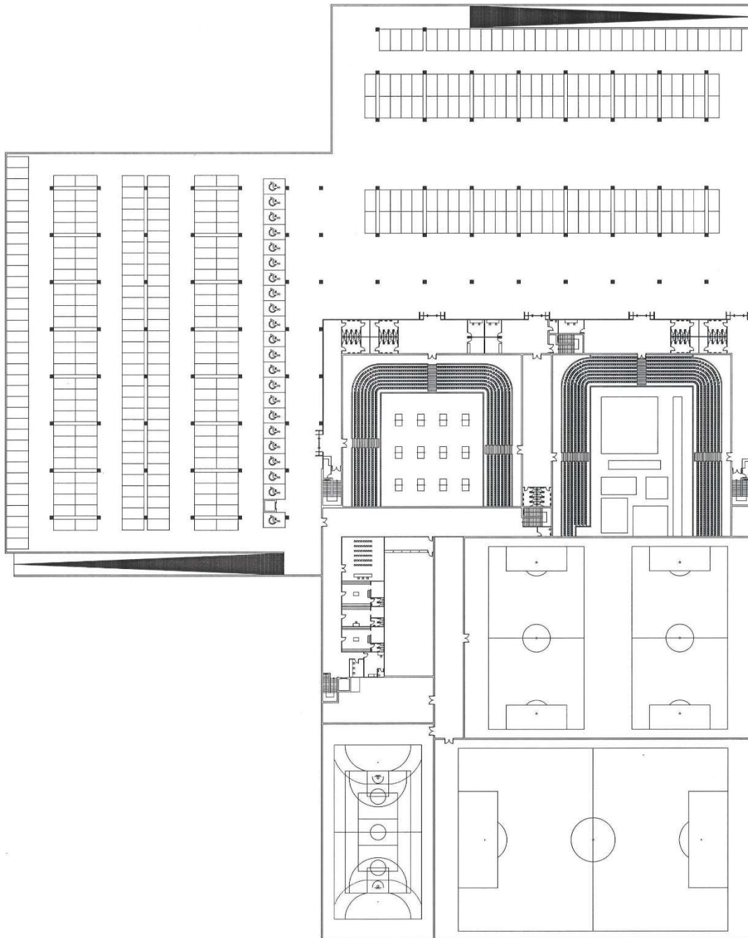
Κάτοψη υπογείου
