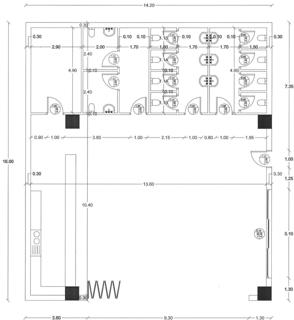
Κάτοψη καταστήματος
