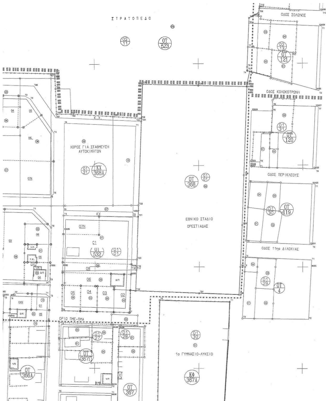
Απόσπασμα ρυμοτομικού σχεδίου
