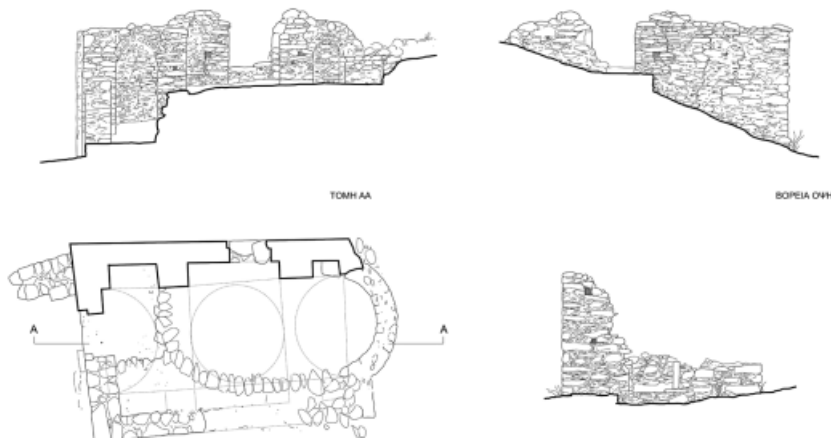
Εικ. 20. Κάστρο Βατίκων. Ναός στα νοτιοδυτικά του κάστρου. Κάτοψη, τομή κατά μήκος, δυτική και βόρεια όψη.
