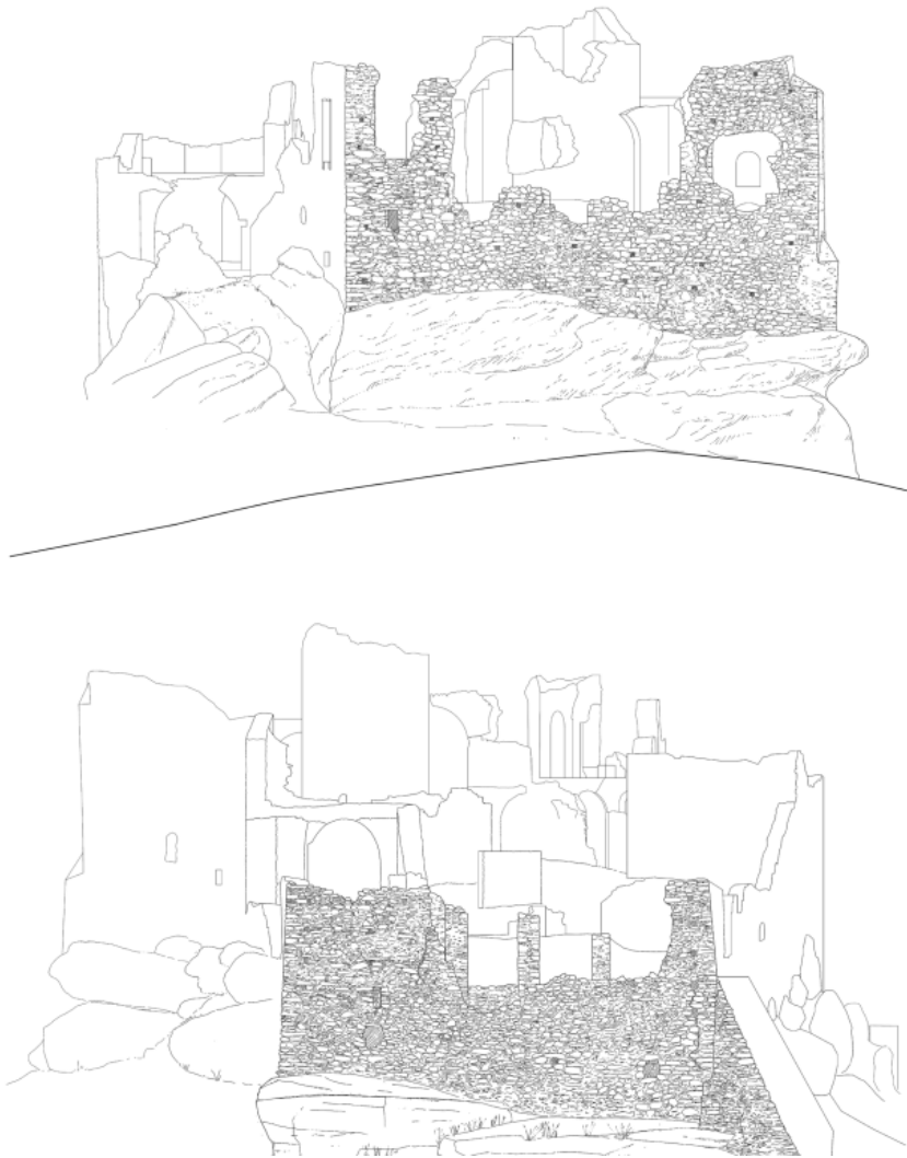
Εικ. 7. Κάστρο Βατίκων. Νότια και Βόρεια όψη του κάστρου.
