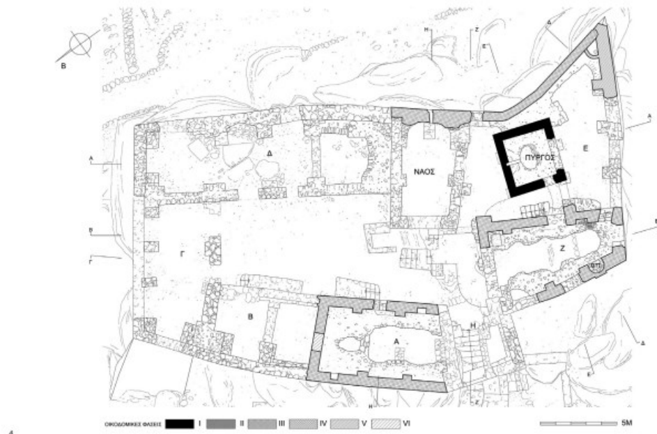
Εικ. 4. Κάστρο Βατίκων. Κάτοψη ισογείου.
