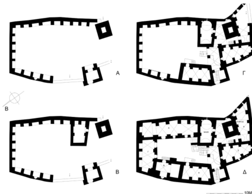
Εικ. 16. Κάστρο Βατίκων. Κάτοψη των ισογείων σε αναπαράσταση στις κύριες οικοδομικές περιόδους.
