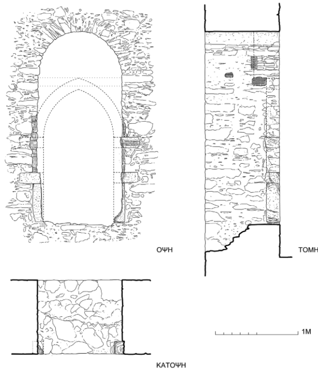
Εικ. 15. Κάστρο Βατίκων. Η κεντρική είσοδος του ναού του Κάστρου.
