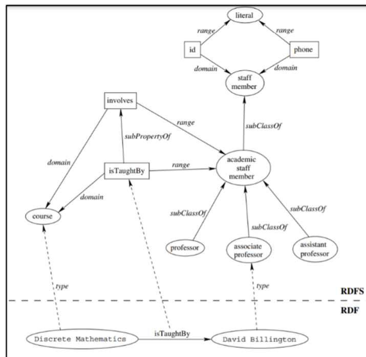
Εικόνα 3. Επίπεδα RDF και RDFS 25
