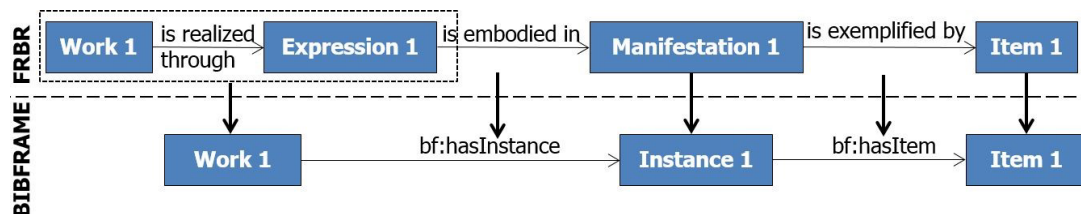
Εικόνα 7. Αντιστοίχιση FRBR με BIBFRAME 2.0 43
