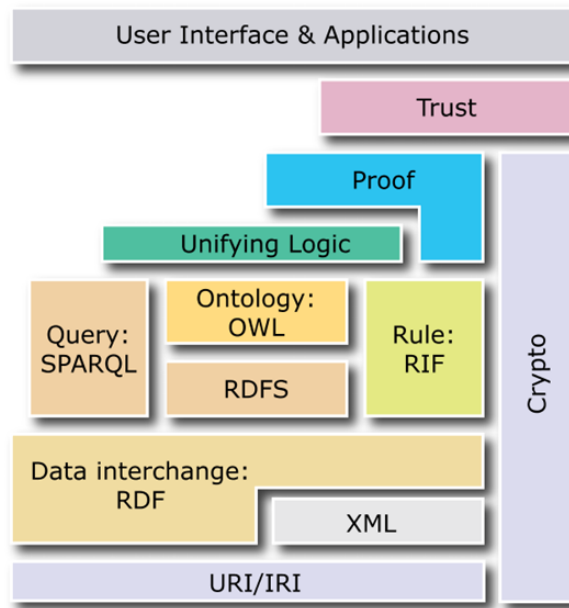
Εικόνα 1. The Semantic Web Stack 2
